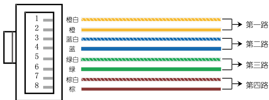
图 2.2-1 RJ45 线序
